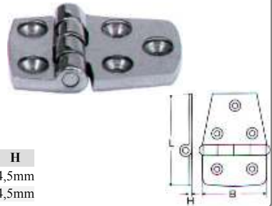
Μεντεσέδες M8429 INOX A4
