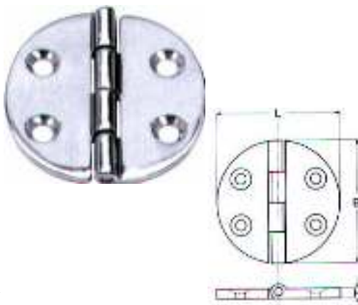
Μεντεσέδες με πύρο M8238 INOX A4
