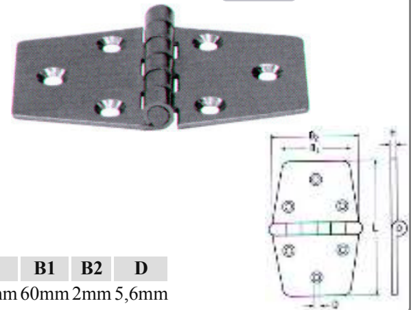
Μεντεσέδες ART1229 INOX A4
