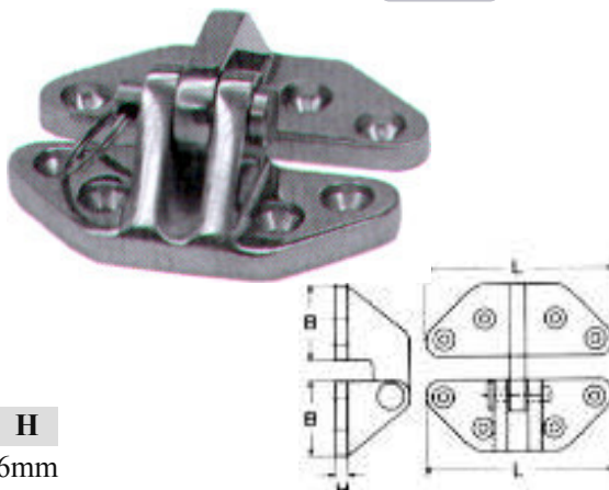
Μεντεσέδες με πύρο M8238 INOX A4
