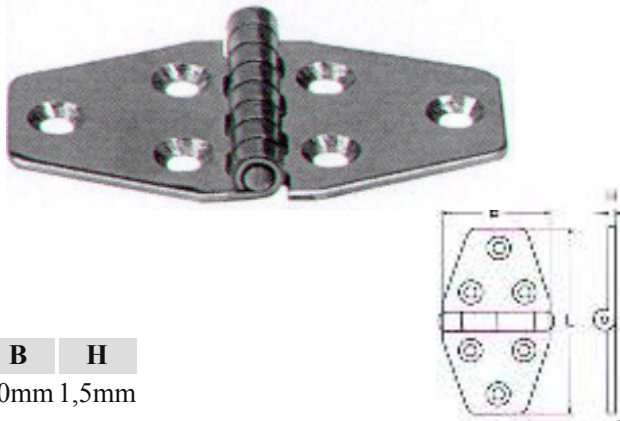
Μεντεσέδες M8151 INOX A4
