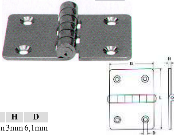
Μεντεσέδες ART1228 INOX A4
