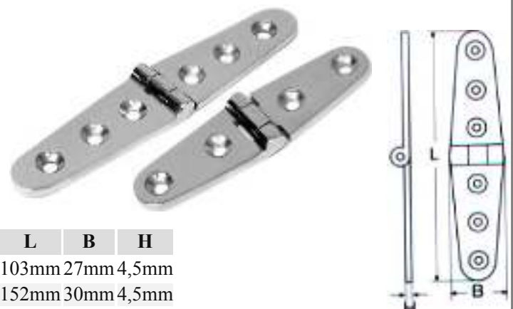
Μεντεσέδες μακρόστενοι M8235 INOX A4
