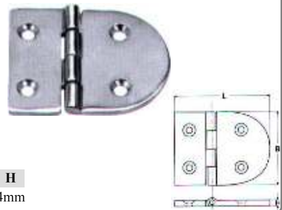
Μεντεσέδες μακρόστενοι M8235 INOX A4
