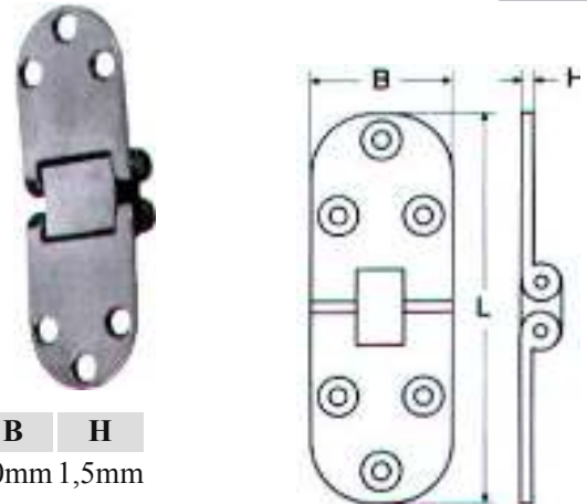
Μεντεσέδες χυτοί M8234 INOX A4
